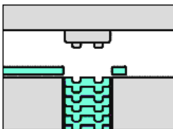
ダボカシメ
