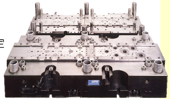
プレス金型 （モーターコアを打ち抜く装置）
